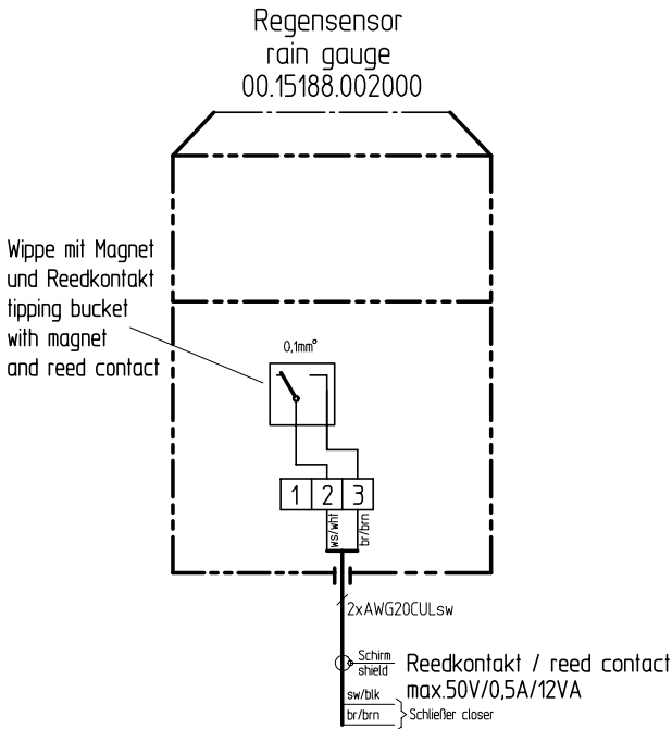
Niederschlags-Sensoren (15188) / (15188 W4)
