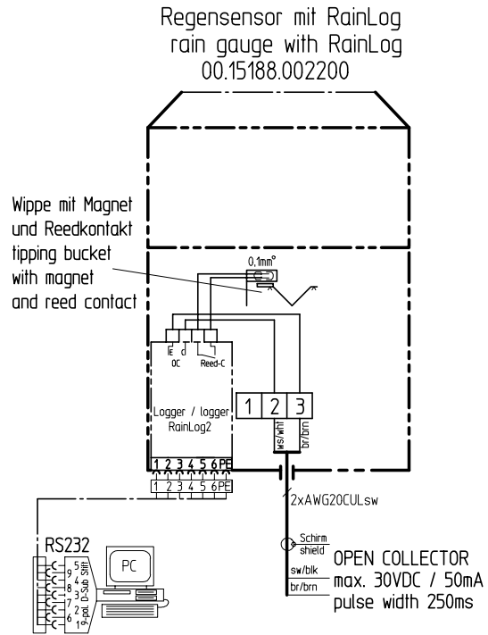
Niederschlags-Sensoren (15188 HD) / (15188 HDW4)
