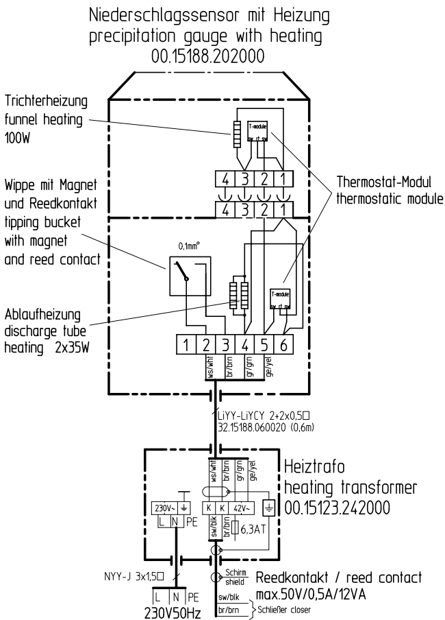
Niederschlags-Sensoren (15188 H) / (15188 HW4)
