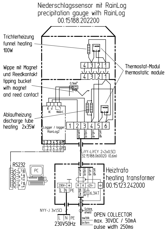
Niederschlags-Sensoren (15188 HD) / (15188 HDW4)
