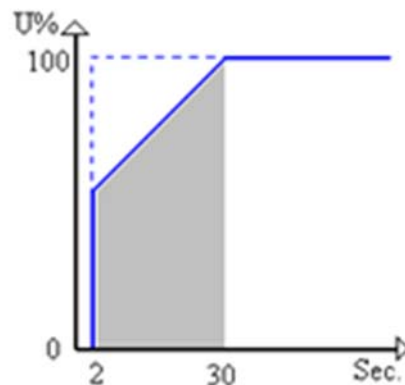
Abbildung 27 Startrampenzeit
