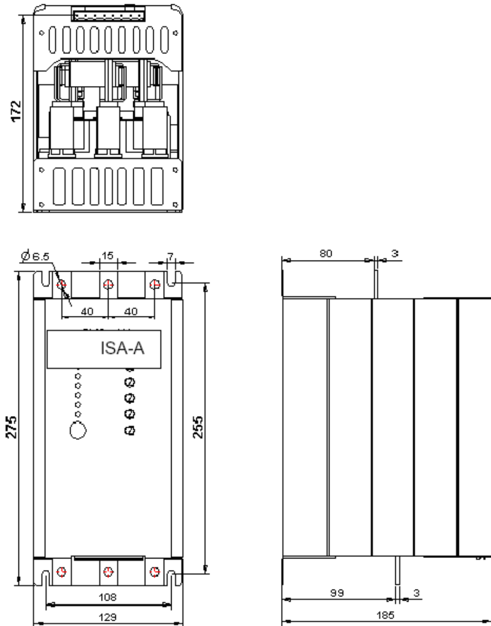
Abbildung 32 Maßzeichnung Gehäuse A2
