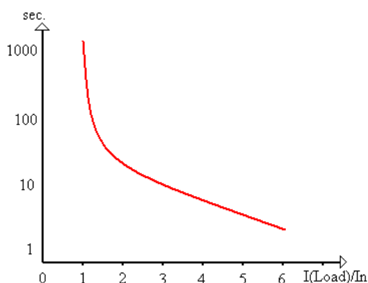
Abbildung 19 Elektronische Überlastauslösung
