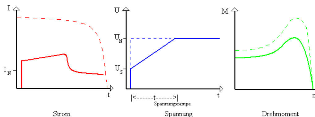
Abbildung 17 Sanft-Start Charakteristika
