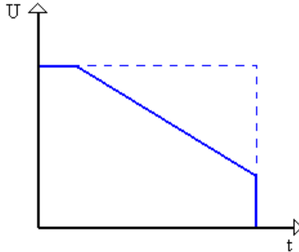
Abbildung 14 Spannungsverlauf Sanftstopp
