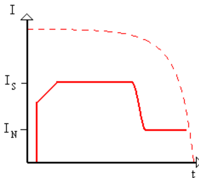
Abbildung 11 Stromverlauf mit Strombegrenzung
