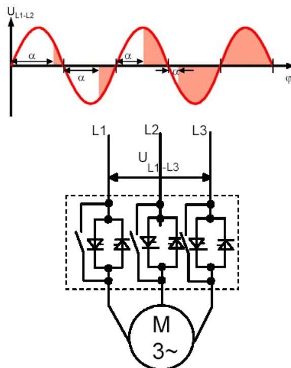
Abbildung 7 Phasenanschnittsteuerung und schematischer Aufbau eines Sanftanlassers
