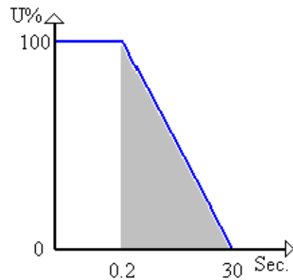
Abbildung 28 Stopprampenzeit
