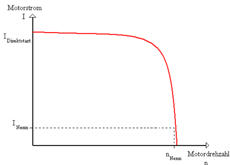
Abbildung 3 Typischer Anlaufstrom eines Asynchronmotors
