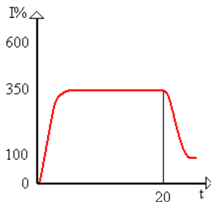
Abbildung 26 Strombegrenzung
