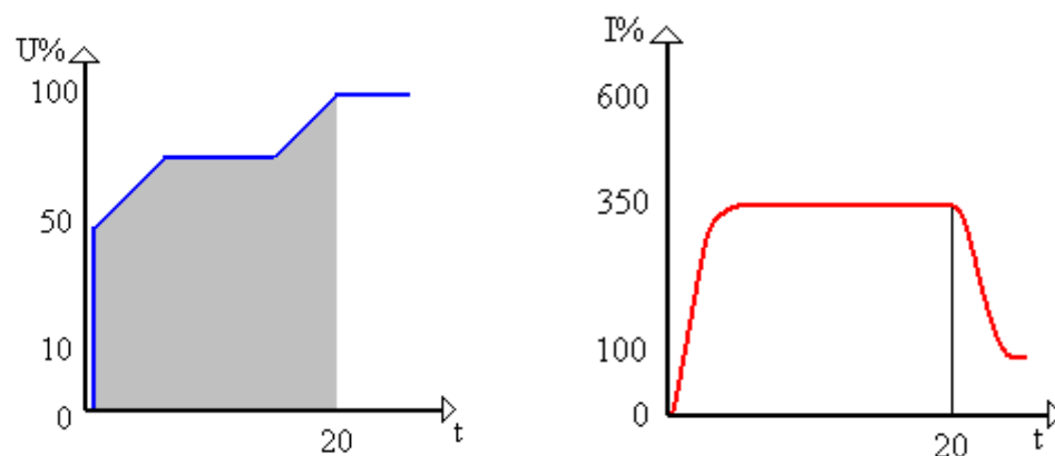
Abbildung 30 Beispiele von Startkurven 2
