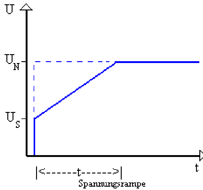
Abbildung 8 Klemmenspannung des Motors
