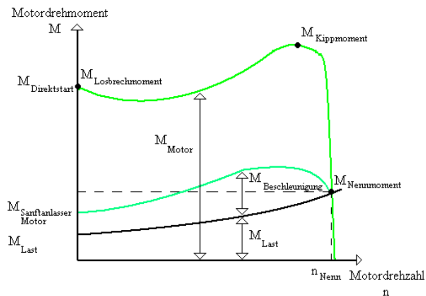
Abbildung 6 Reduziertes Anlaufdrehmoment des Asynchronmotors
