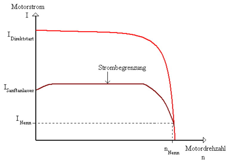
Abbildung 5 Reduzierter Anlaufstrom des Asynchronmotors
