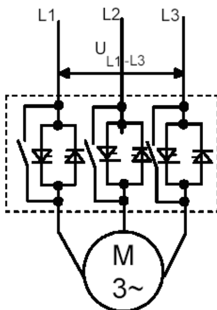
Abbildung 21 Bypass- Kontakte
