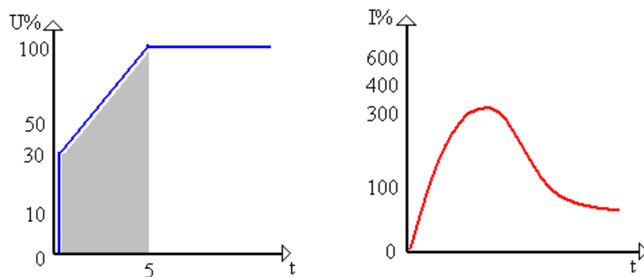
Abbildung 29 Beispiele von Startkurven
