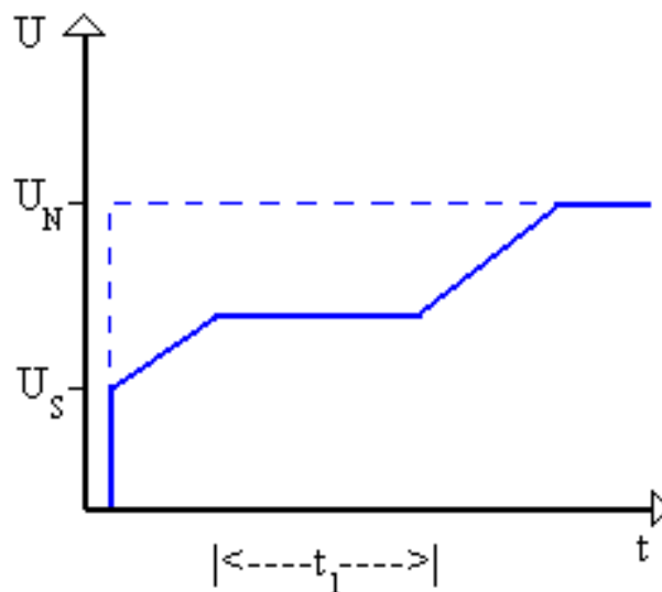
Abbildung 10 Klemmenspannung des Motors mit Strombegrenzung
