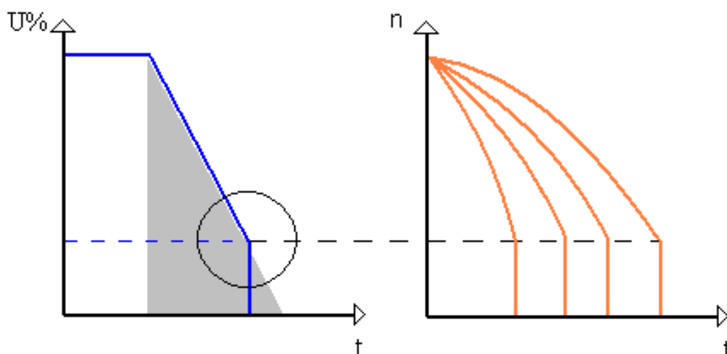
Abbildung 16 Sanftstopp mit Pumpenkurven
