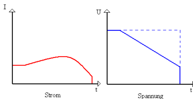
Abbildung 18 Sanft-Stopp Charakteristika
