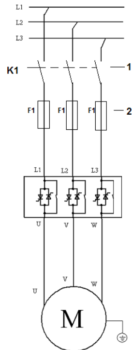
Abbildung 22 Schaltbild
