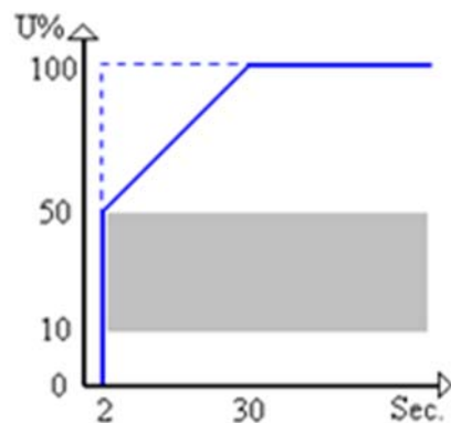
Abbildung 25 Startmoment
