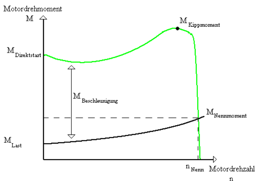
Abbildung 4 Typisches Anlaufdrehmoment eines Asynchronmotors
