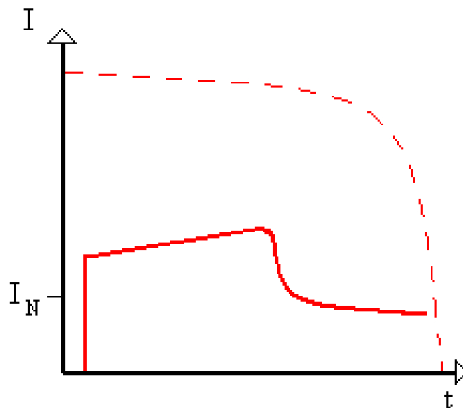
Abbildung 9 Stromverlauf
